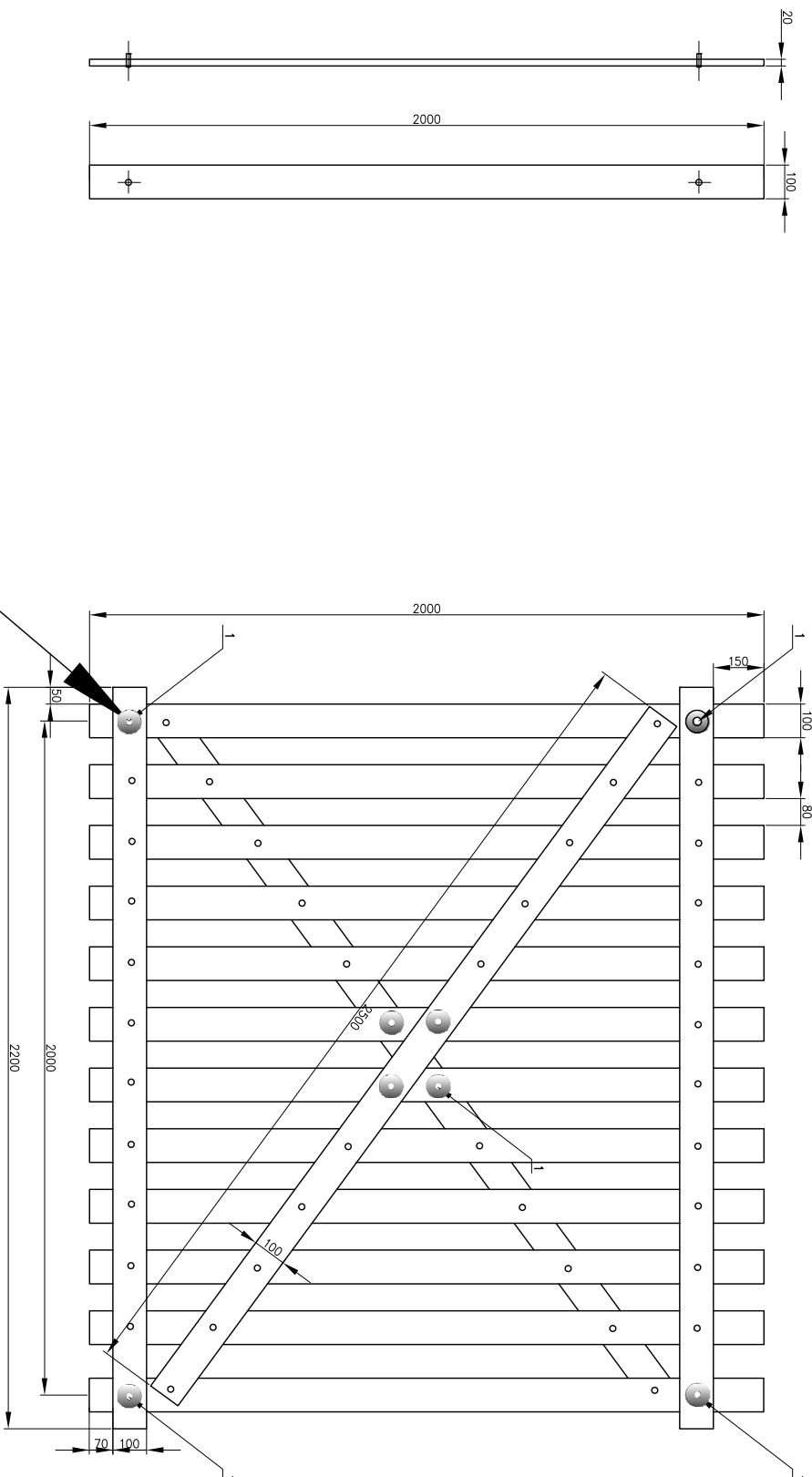
DETAILED VIEW ДЕТАЛЬНЫЙ ВИД
